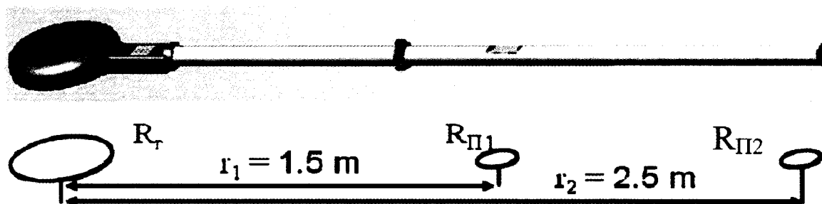
Рисунок 1 Схема аппаратуры ЭМС.
