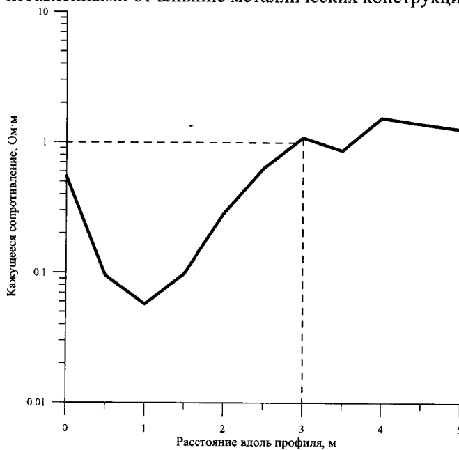
Рисунок 6 Профильная кривая кажущегося сопротивления, построенная для тестового объекта «Свая». Тело сваи располагается в точке 1 м по профилю.
